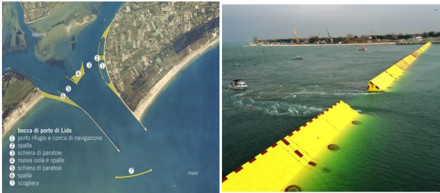
صورة (8): توضح استخدام الحواجز في مواجهة الفيضانات في مدينة البندقية
