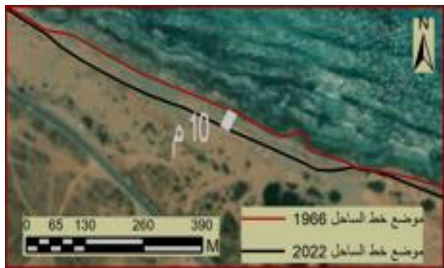
الشكل (9) الجزء الشرقي لخط الساحل لمدينة لبدة (شرق مصب وادي لبدة)
