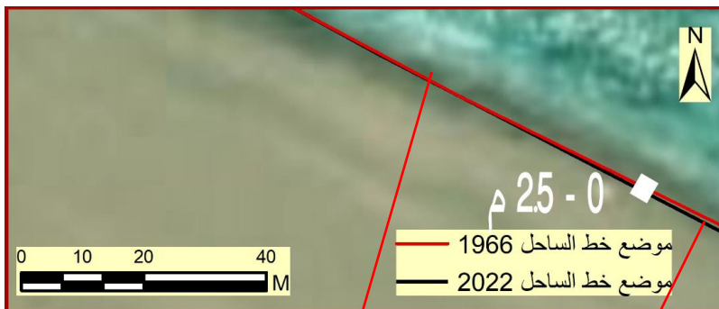
الشكل (9) خط الساحل بالجزء الغربي لمدينة لبدة الأثرية
