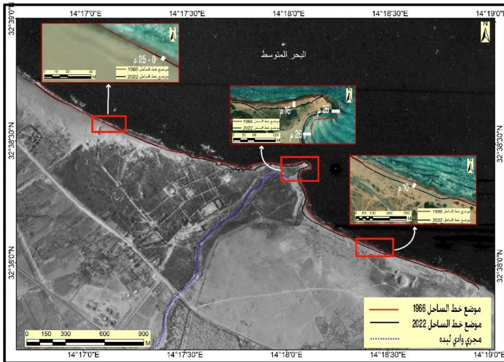
الشكل (8) تغير خط الساحل من سنة 1966-2022م.
